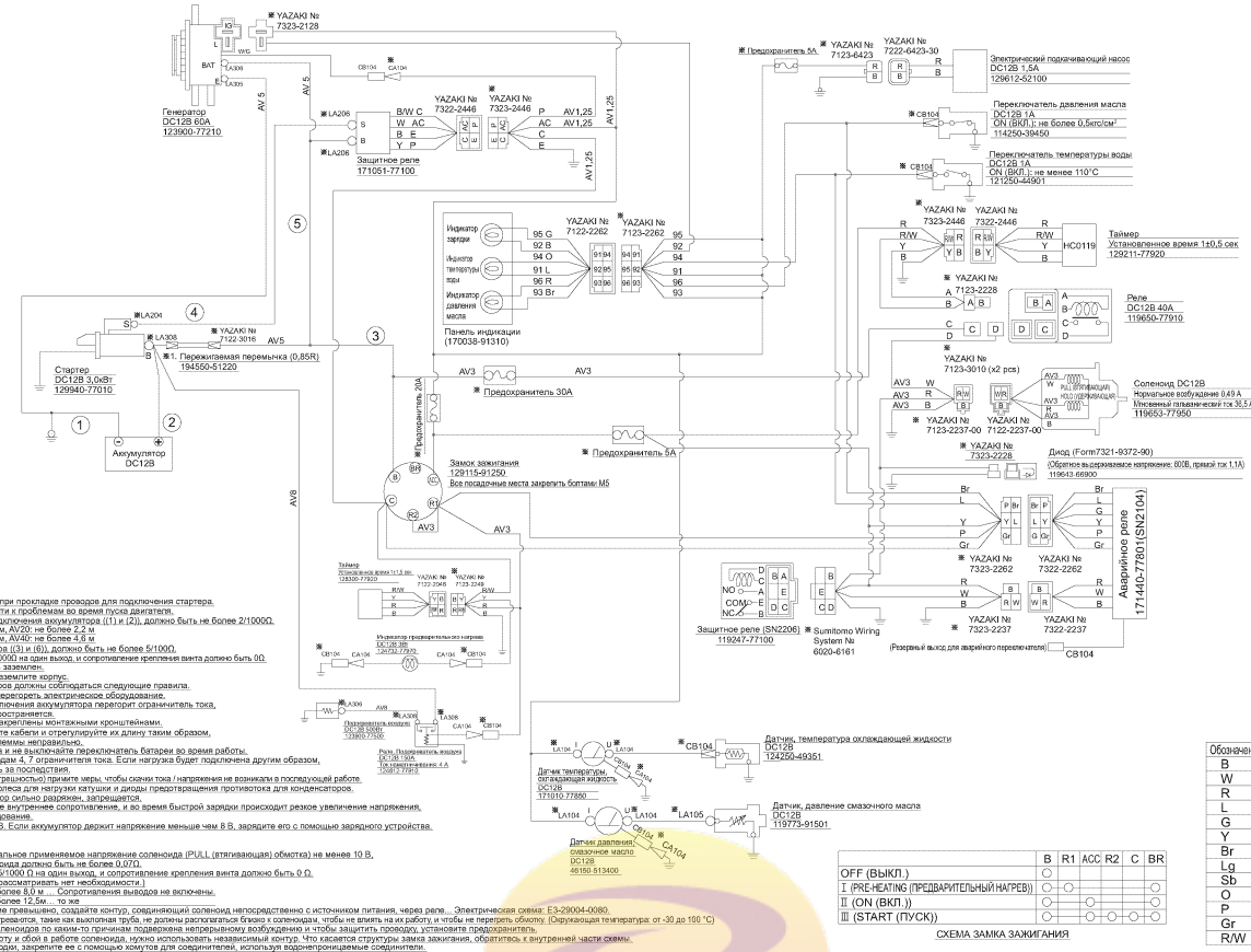
СХЕМА ЗАМКА ЗАЖИГАНИЯ
